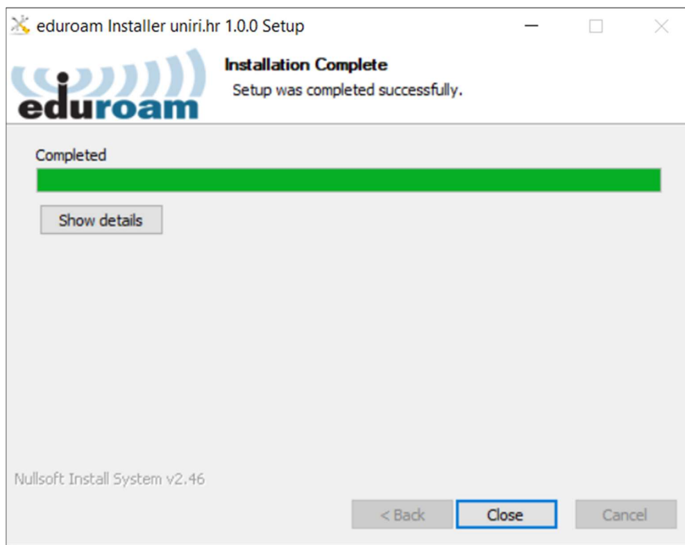
Slika 8. Završetak instalacije
