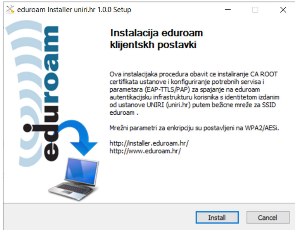
Slika 5. Pokretanje instalacije
